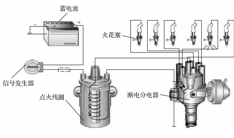
图 1-11 汽油机点火系统组成
