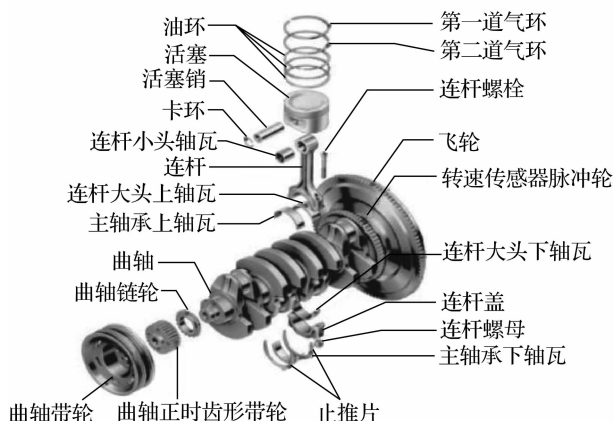
图 1-7 曲柄连杆机构的组成
