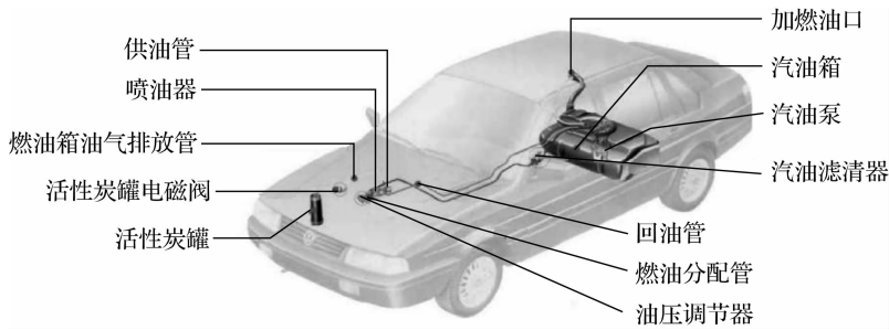
图 1-9 汽油机燃油系统
