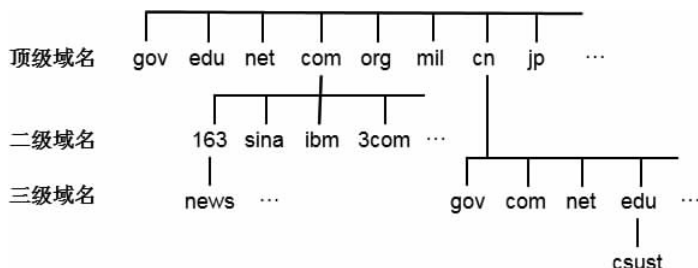
图 2-27 DNS 层次结构示意图
