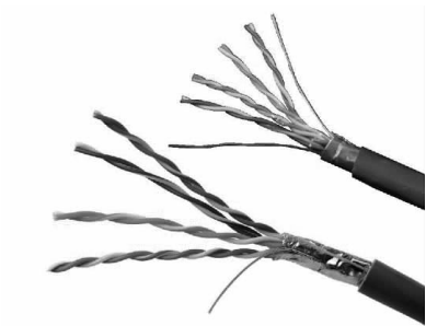
图 2-7 屏蔽双绞线
