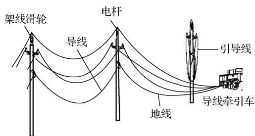
图 2-3 低压电力线路的结构
