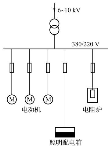
图 2-4 低压电力线路的接线
