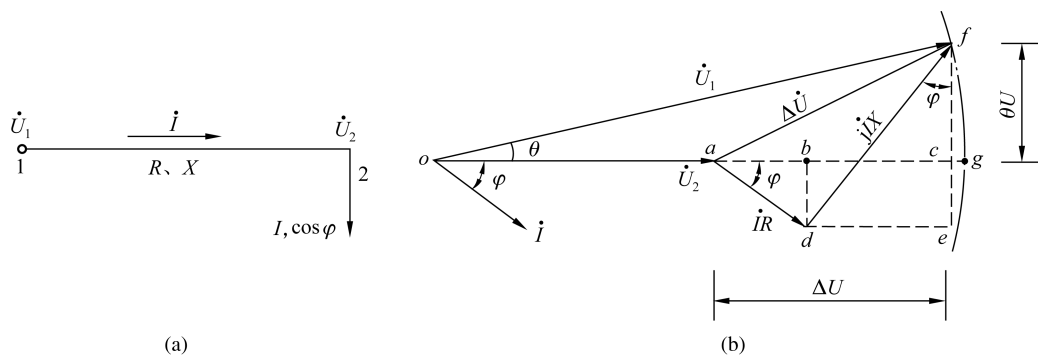
图 1-24 计算线路上的电压降和电压损失
