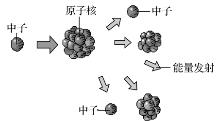
图 1-10 核裂变过程
