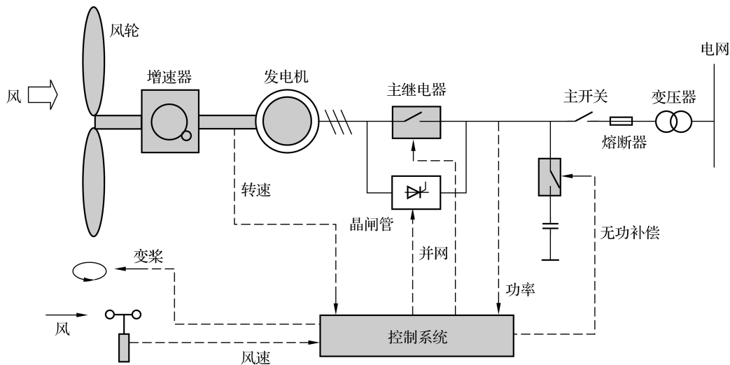
图 1-12 风力发电的结构和原理
