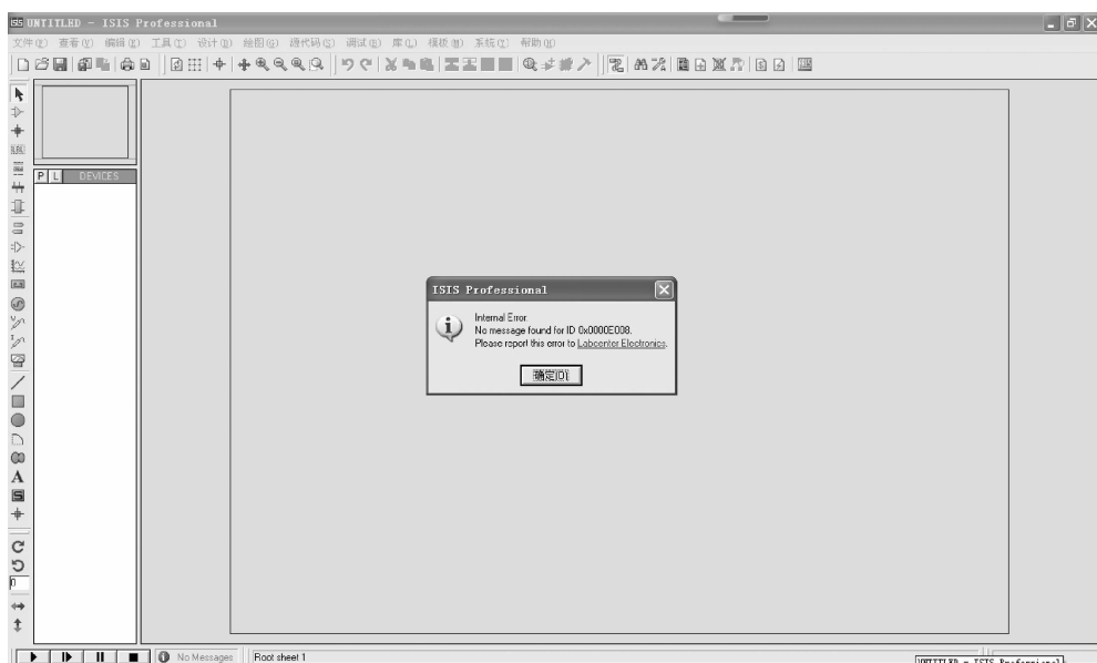
图 2-9 绘图前界面 2
