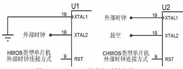
图 2-4 AT89C51 的外部时钟电路
