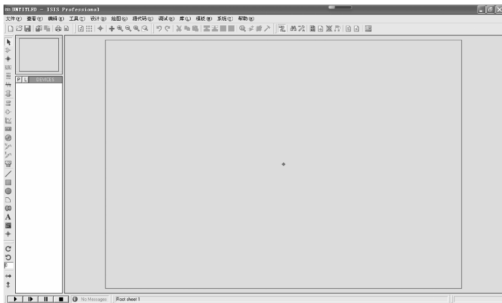
图 2-10 绘图界面
