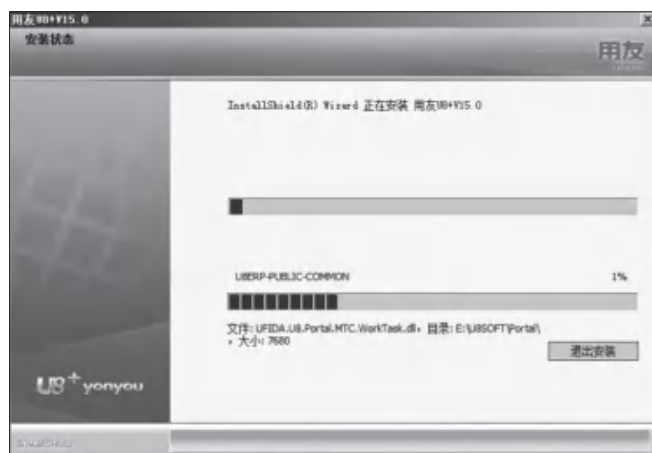
图 1-24 安装界面
