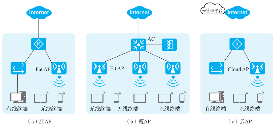
图 1-9 无线接入点
