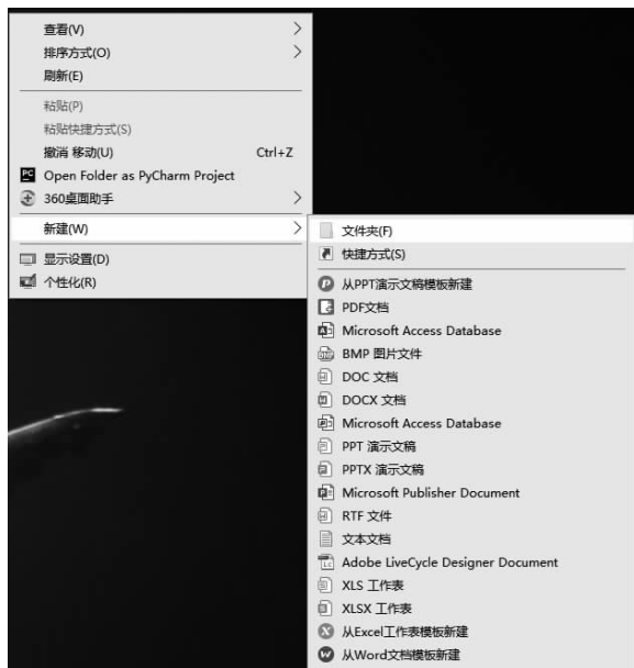
图 1-5-1 新建文件夹
