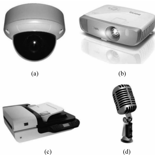
图 1-3-2 外围设备
