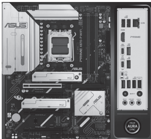
图 1-8 某品牌主板
