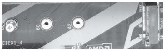
(a) M.2-NVMe 硬盘接口
